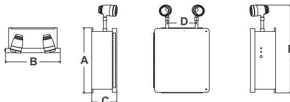
Dimensions (in,mm.)
